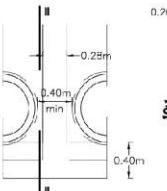
SEMICORTE I-I
